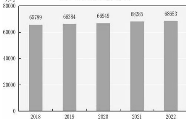
图8 2018-2022年粮食产量
